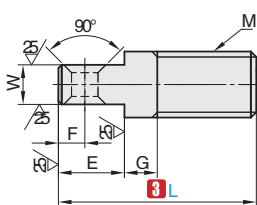
GTKAB GTKBB 两平面型
