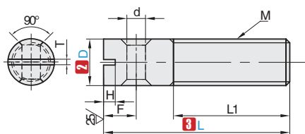
GTKAA GTKBA 直柱型
