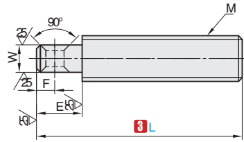
GTKAE GTKBE 全螺纹型
