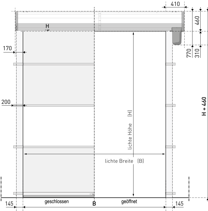
[ Vorderansicht ]
