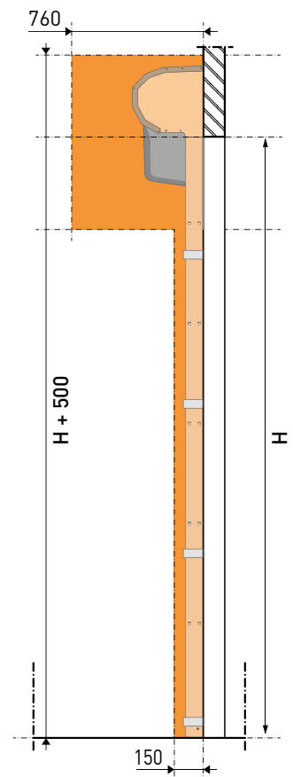
[ Leiterquerschnitt ]
