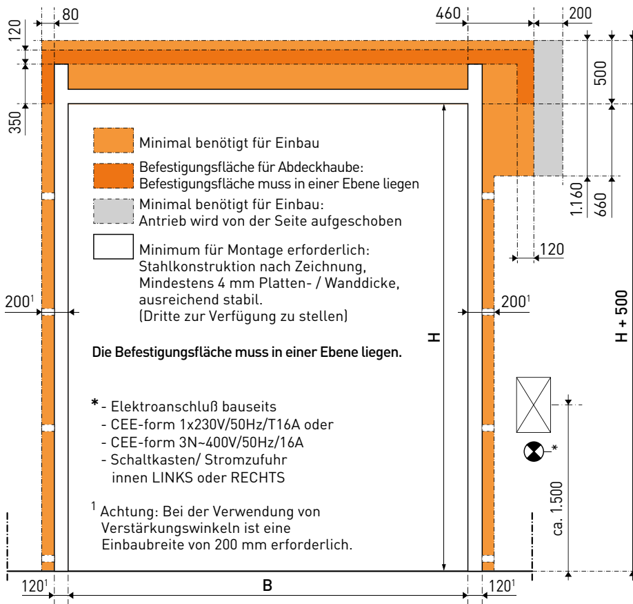
[ Vorderansicht ]
