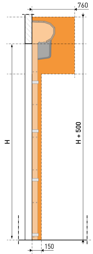
[ Leiterquerschnitt ]
