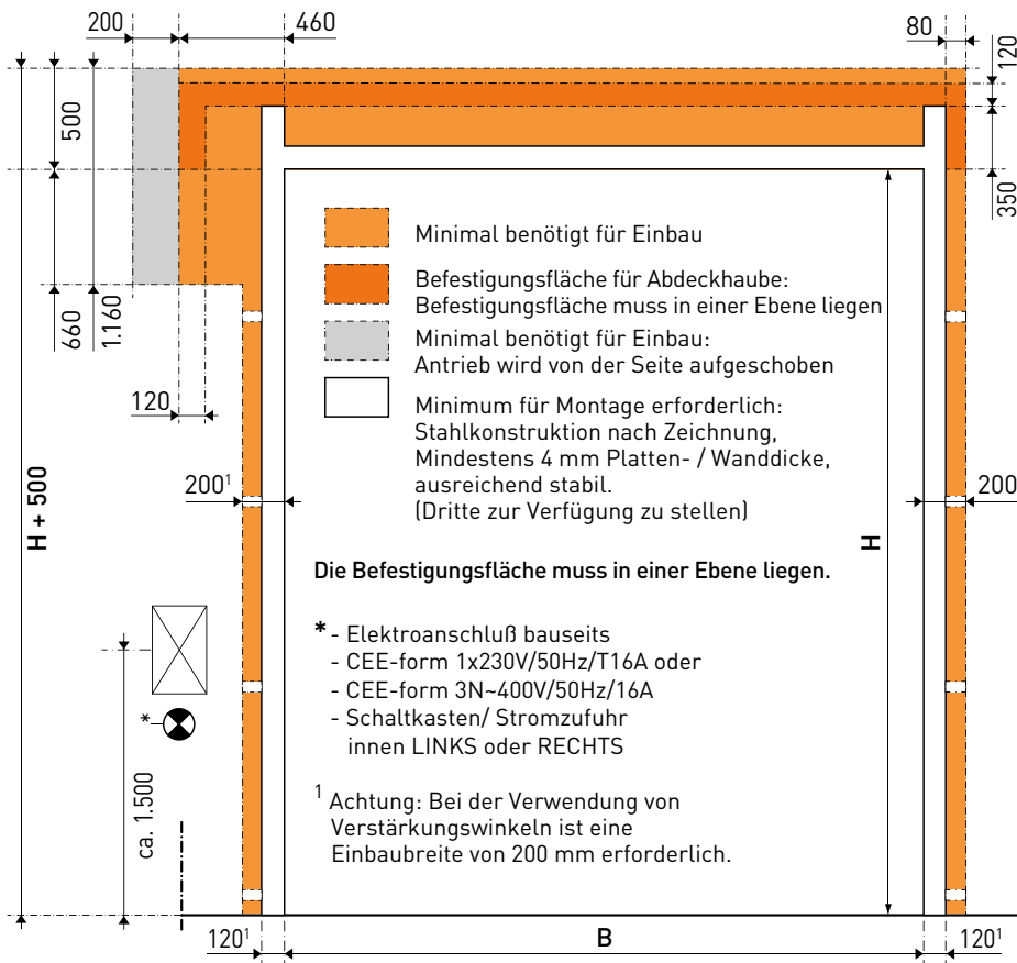
[ Antriebsseite ]
