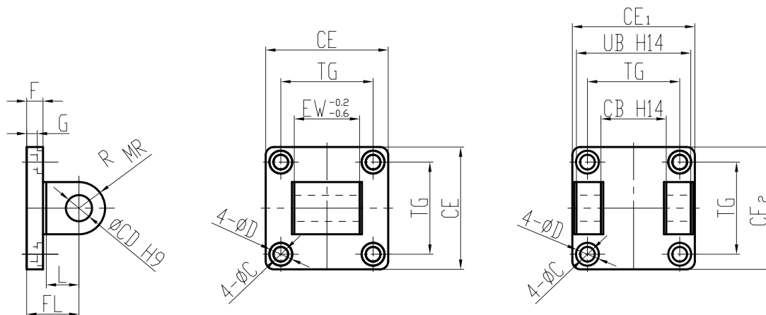
双耳环支架带轴销、平垫片、开口销
