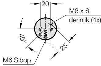
Görünüm X
