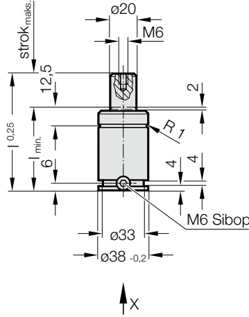
Görünüm X
