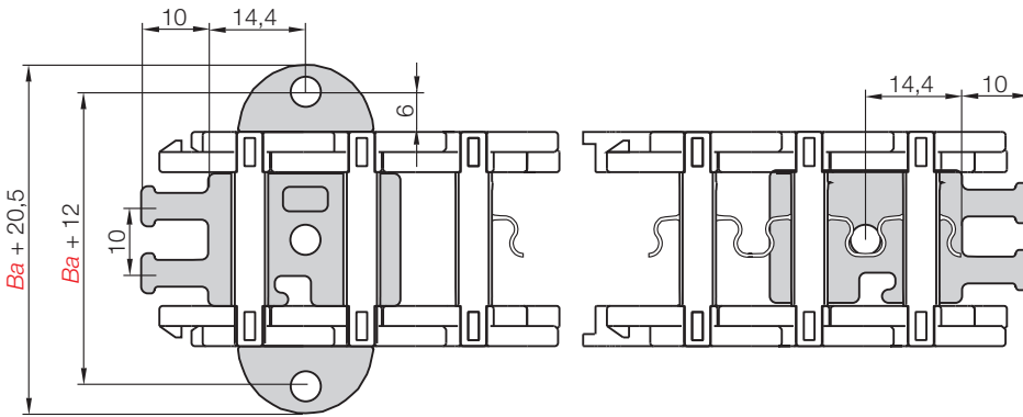
E3.10.....2 Fixed end
