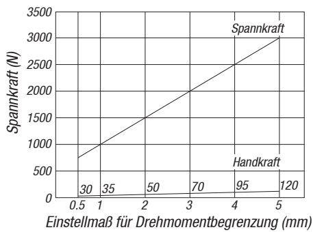
Niederzugspanner 04565-0500 Niederzugspanner 04565-0501
