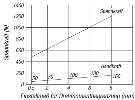
Schwenkspanner 04366-...4540
