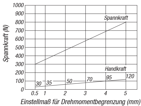
Schwenkspanner 04366-...3232
