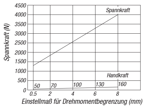
Niederzugspanner 04565-0800 Niederzugspanner 04565-0801
