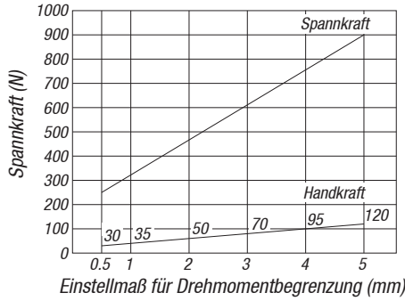
Zugspanner 04400-3240...
