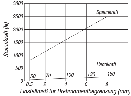
Zugspanner 04400-4050...
