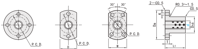
●圆法兰型
