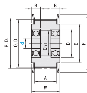
● 两侧轴承型
