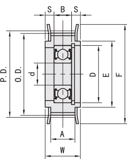
● 中心轴承型-单轴承
