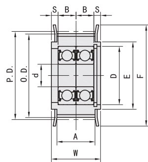
● 中心轴承型-双轴承
