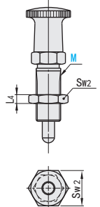
带锁紧螺帽 ZS53S ZS53SE
