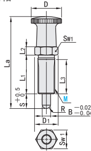
带锁紧螺帽 ZS53S ZS53SE
