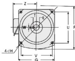
备注: A1 三相马达尺寸; A2 三相刹车马达尺寸
