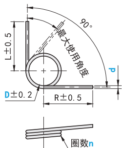
臂角90°
