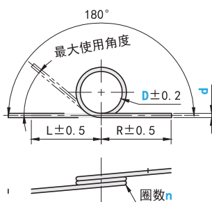
臂角180°
