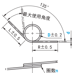
臂角135°
