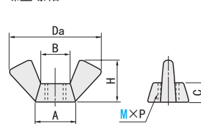
蝶型螺帽
