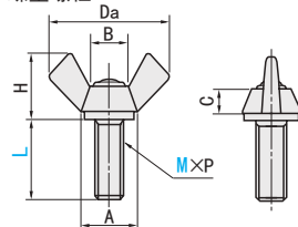
蝶型螺栓
