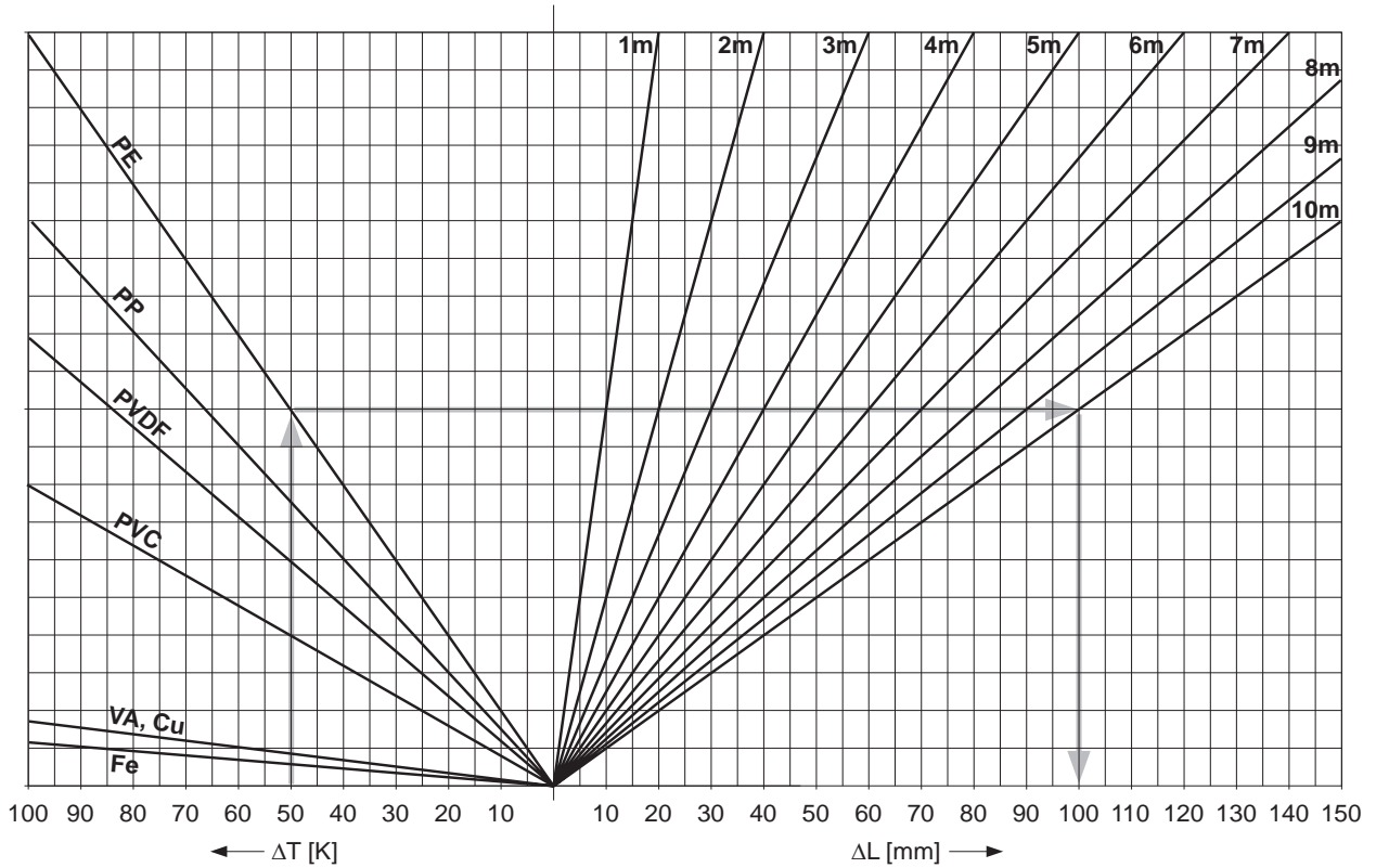
Grafische Bestimmung der Längenänderung
